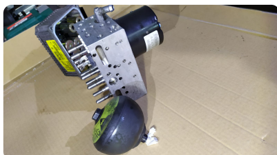
Ремонт блока SBC.
