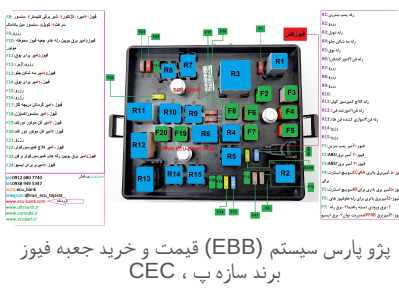
فروشگاه - CEC جعبه فیوز داخل اتاق پژو پارس بزرگ رایان ایسیو
